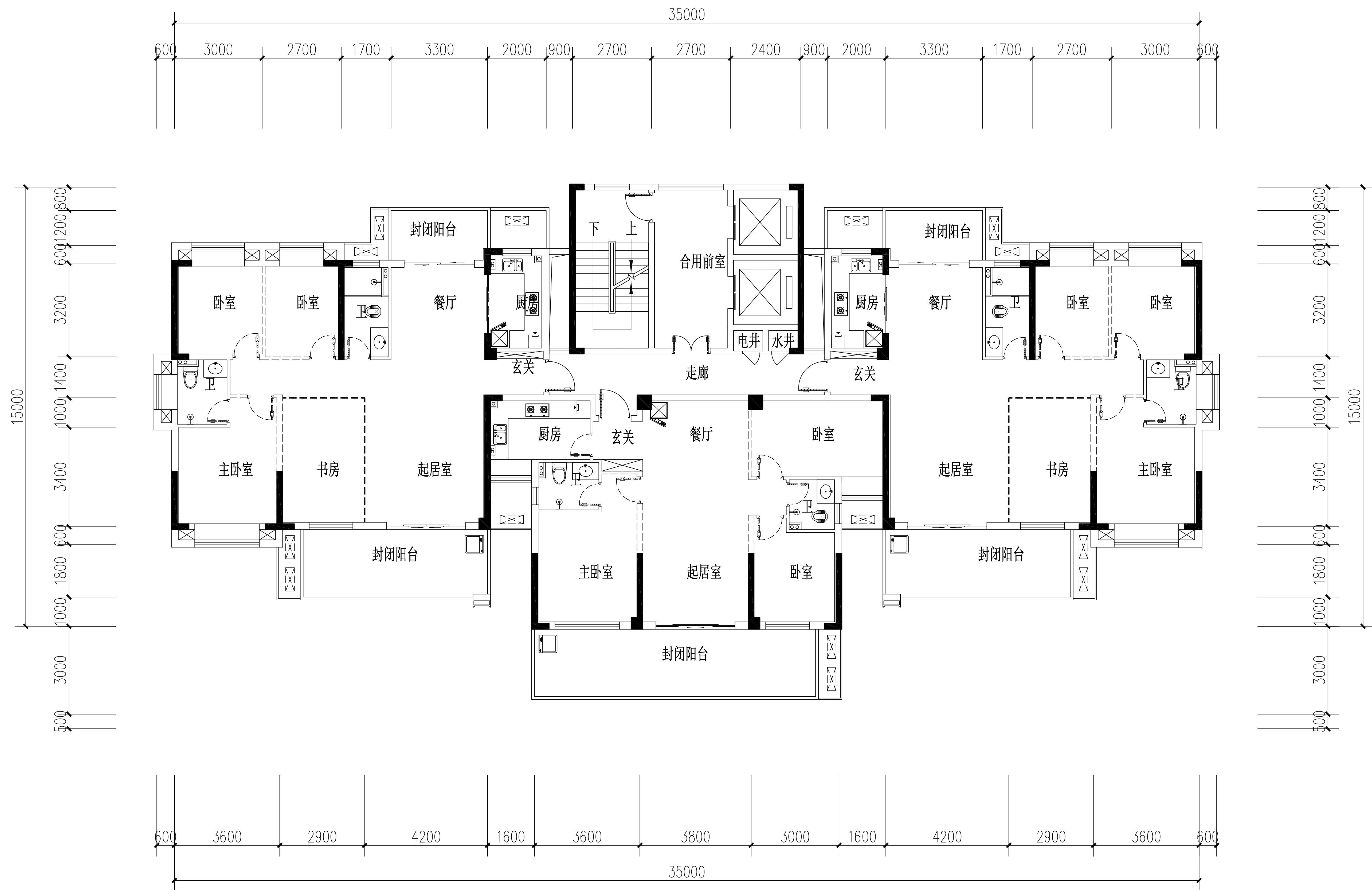
16、18#楼三至十七层平面图1:150
