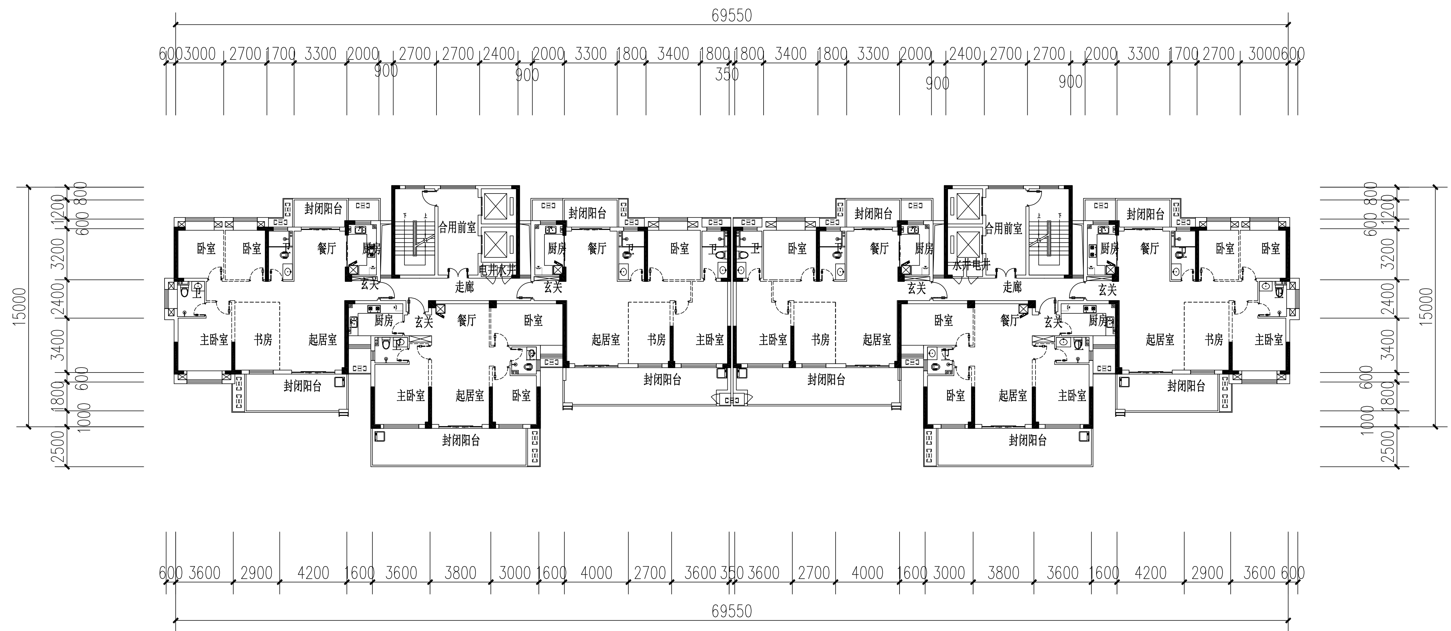
17#楼三至十七层平面图1:300
