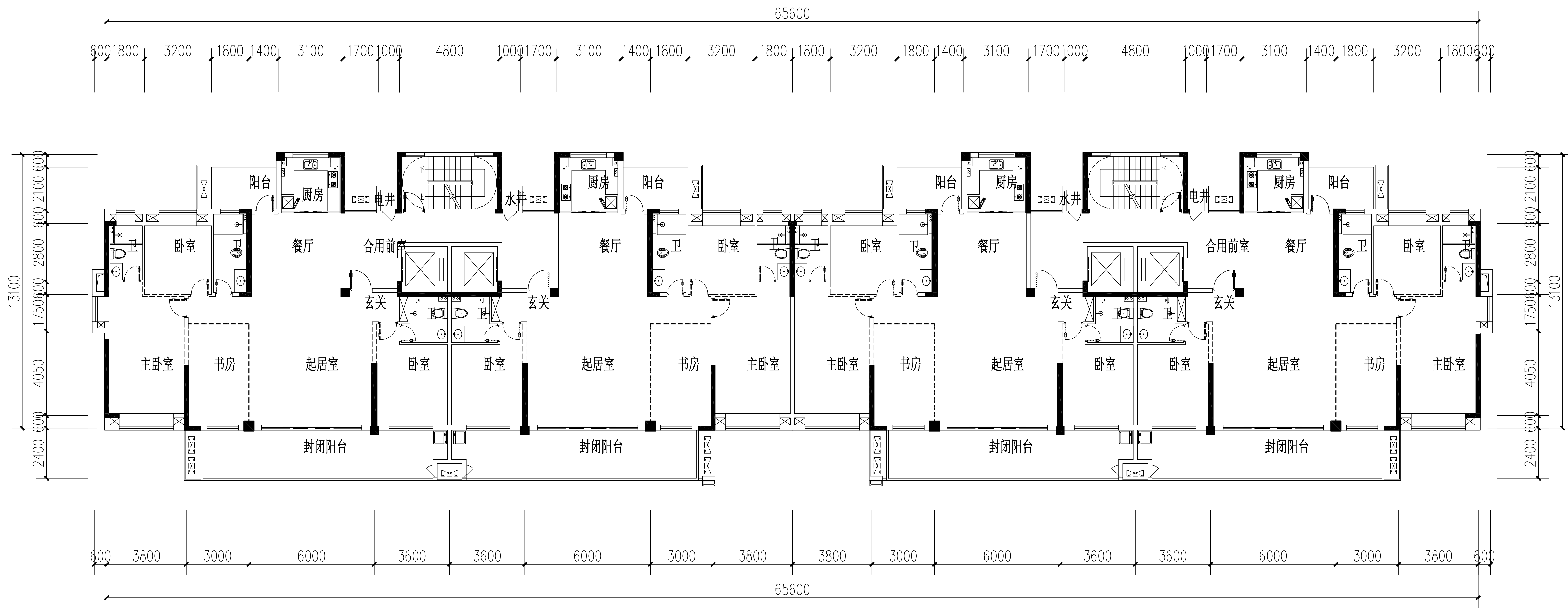
2#三至十七层平面图1:200
