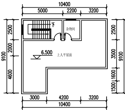
三层平面图 1:200
