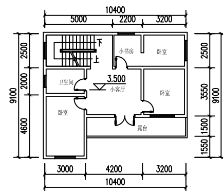
二层平面图 1:200
