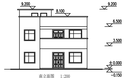
南立面图 1:200
