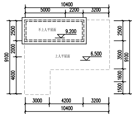
屋顶平面图 1:200
