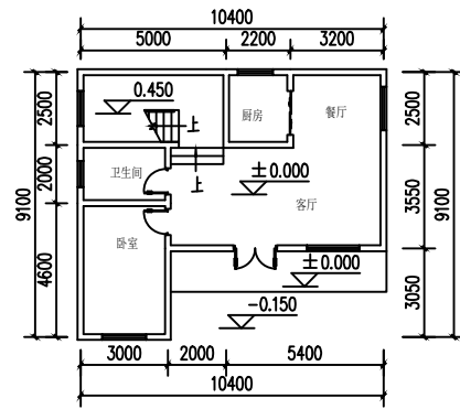
一层平面图 1:200
