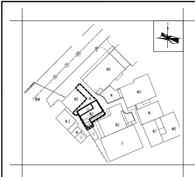
平面位置图 1:500
