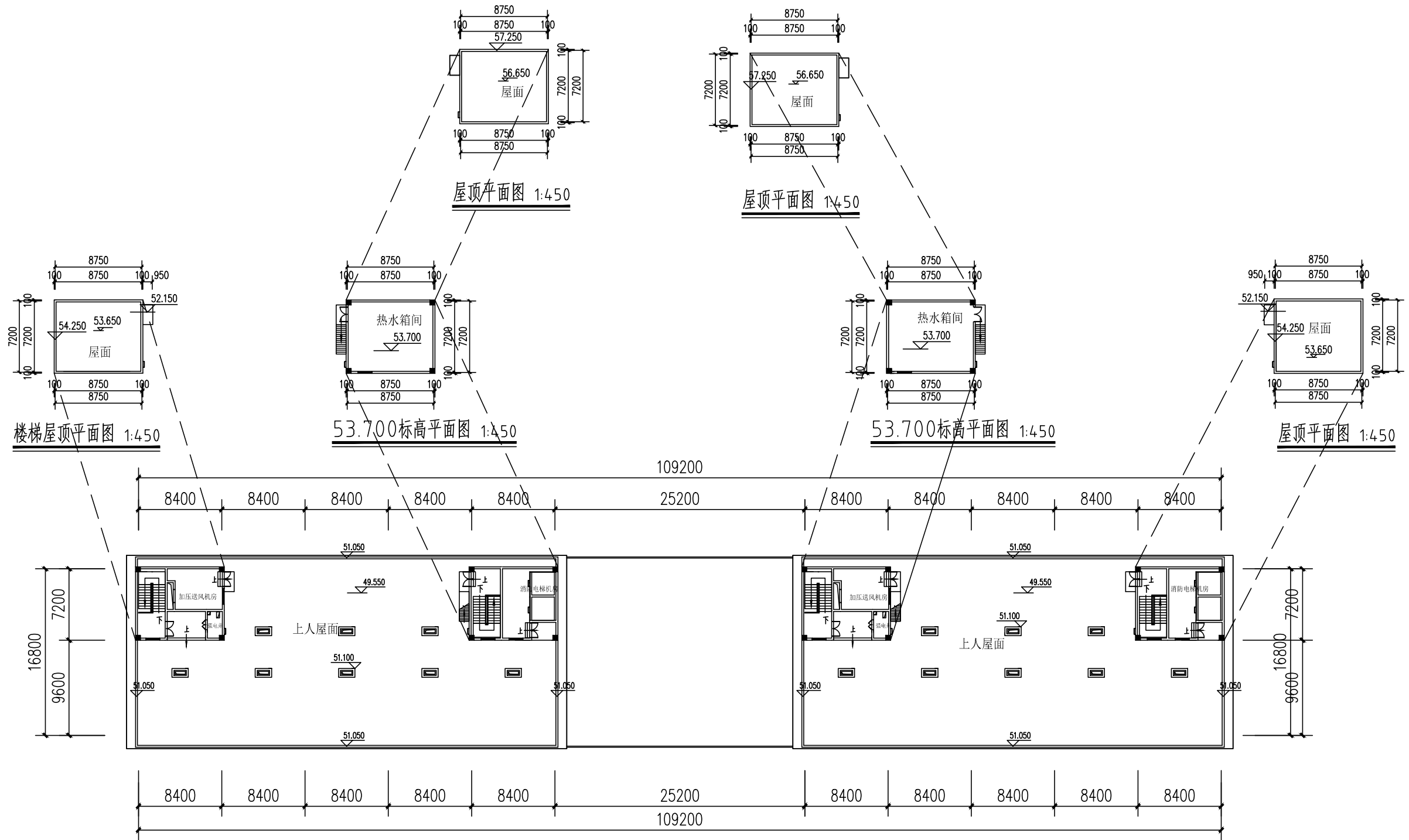
屋顶层平面图 1:450
