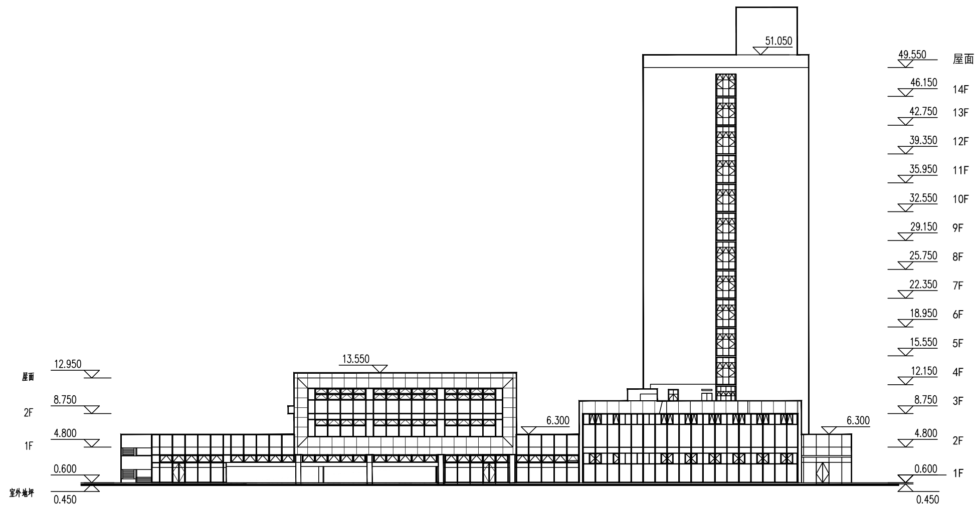
东立面图 1:450
