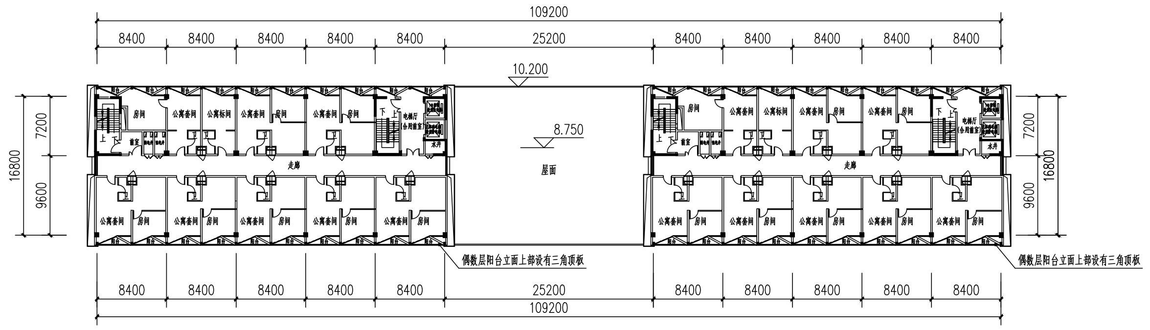
十四层平面图 1:450
