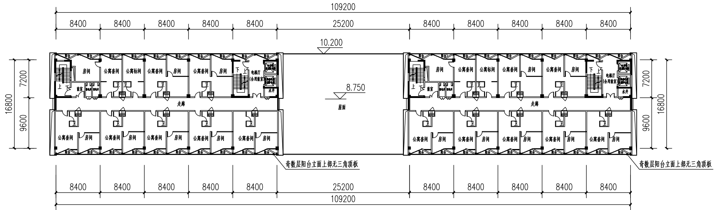
十三层平面图 1:450
