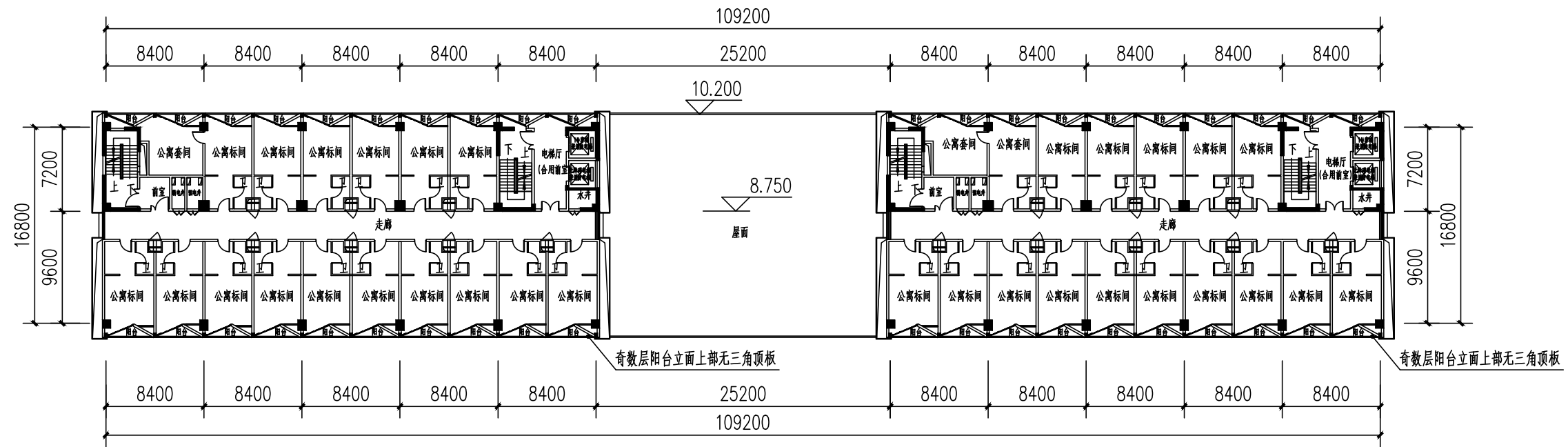
四层至十二层奇数层平面图 1:450
