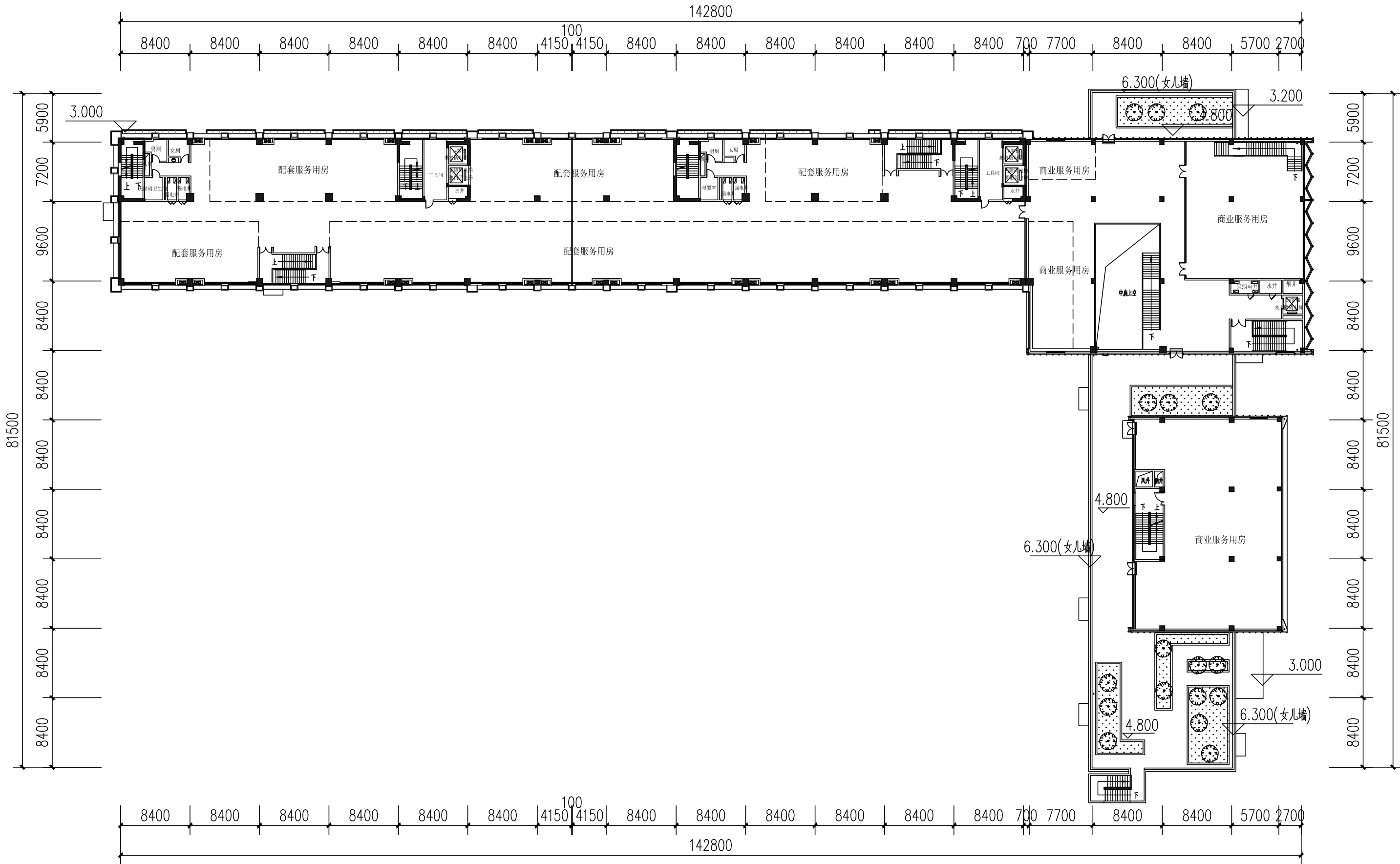
二层平面图 1:450
