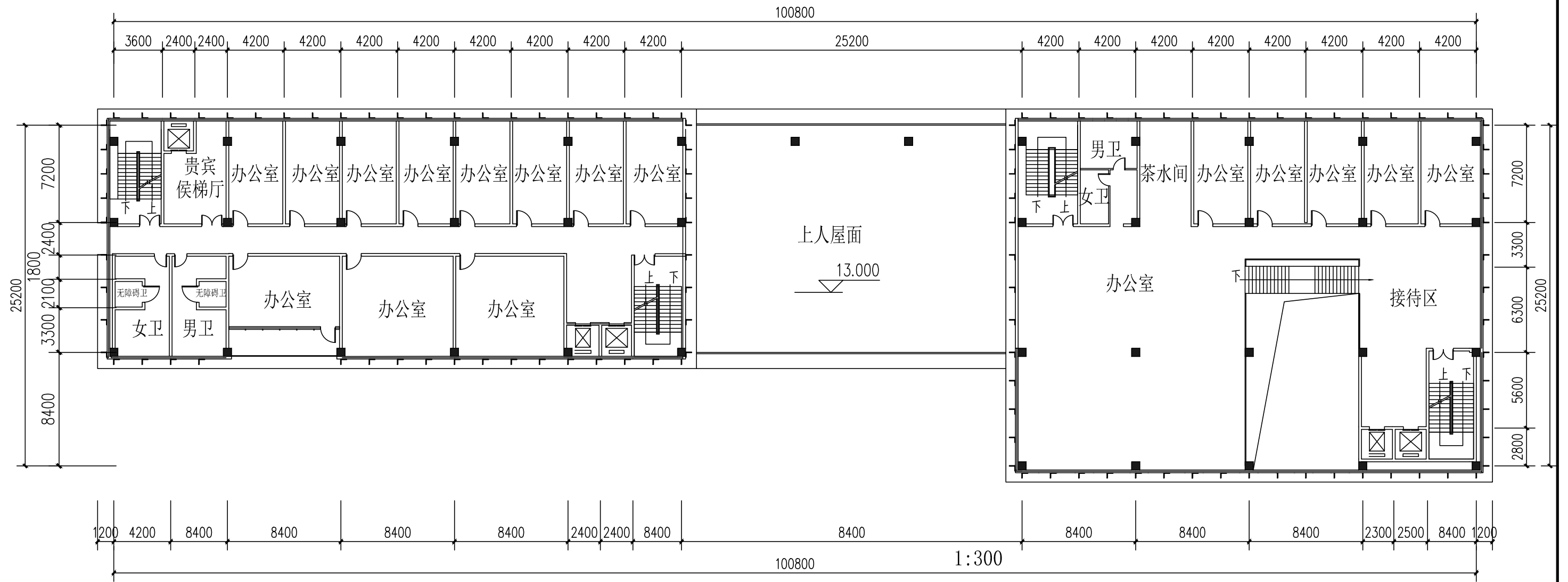
七层平面图 1:300
