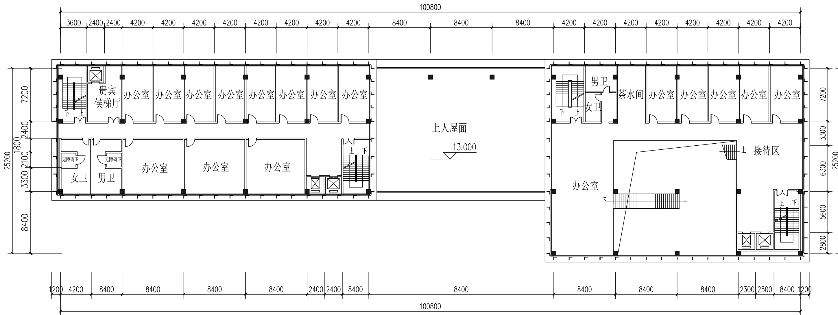
六层平面图 1:300
