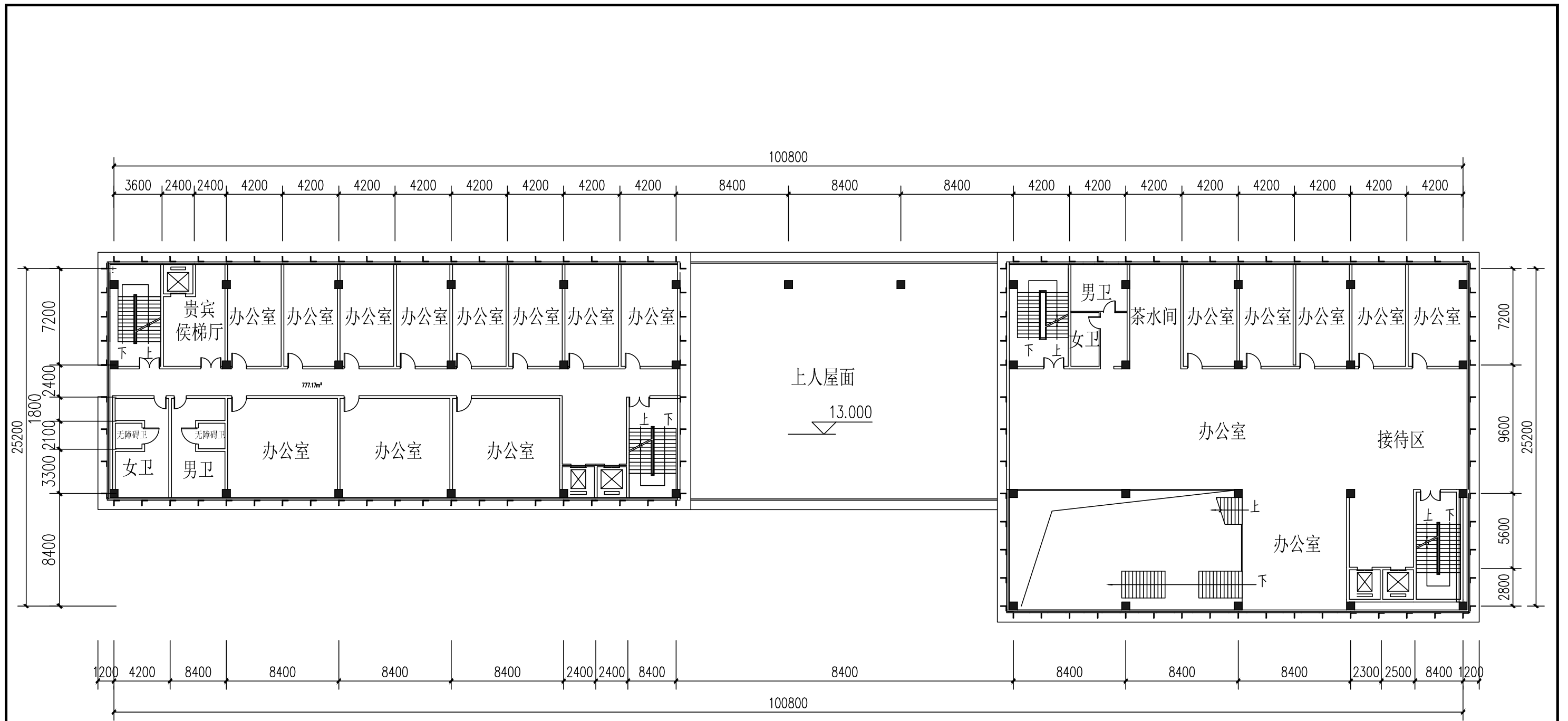
五层平面图 1:300
