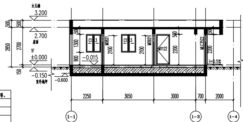
1-1 剖面图 1:100
