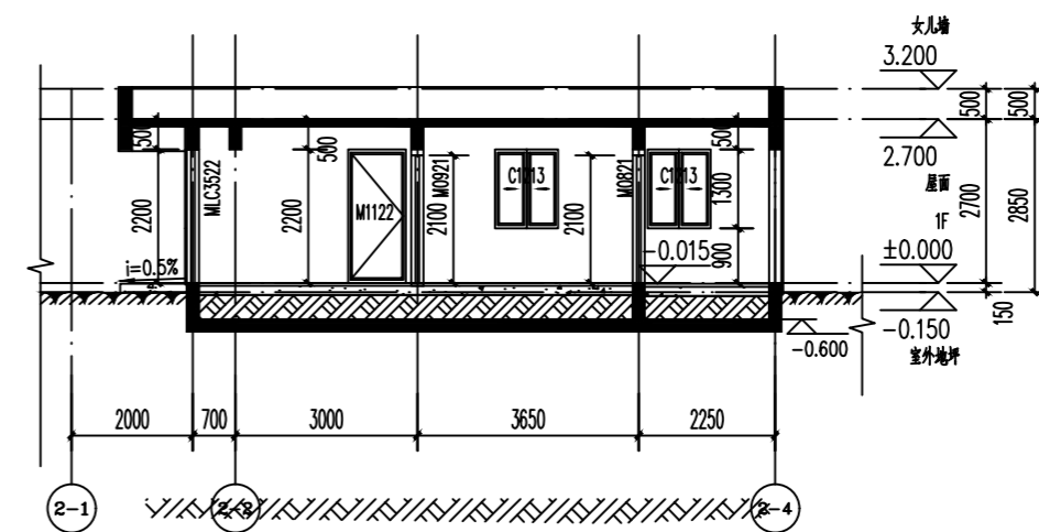
2-2 剖面图 1:100
