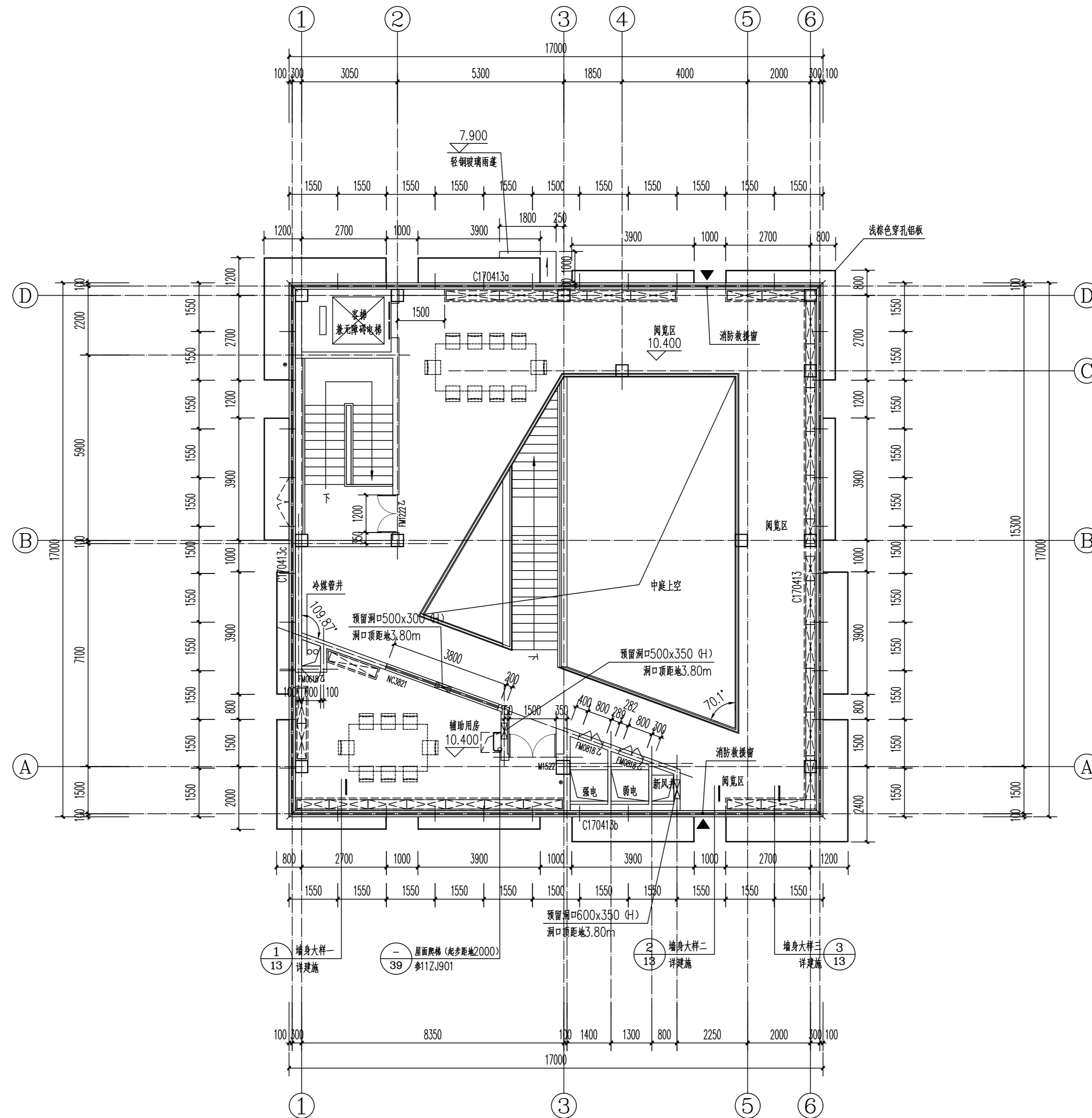
三层平面图 1:100
