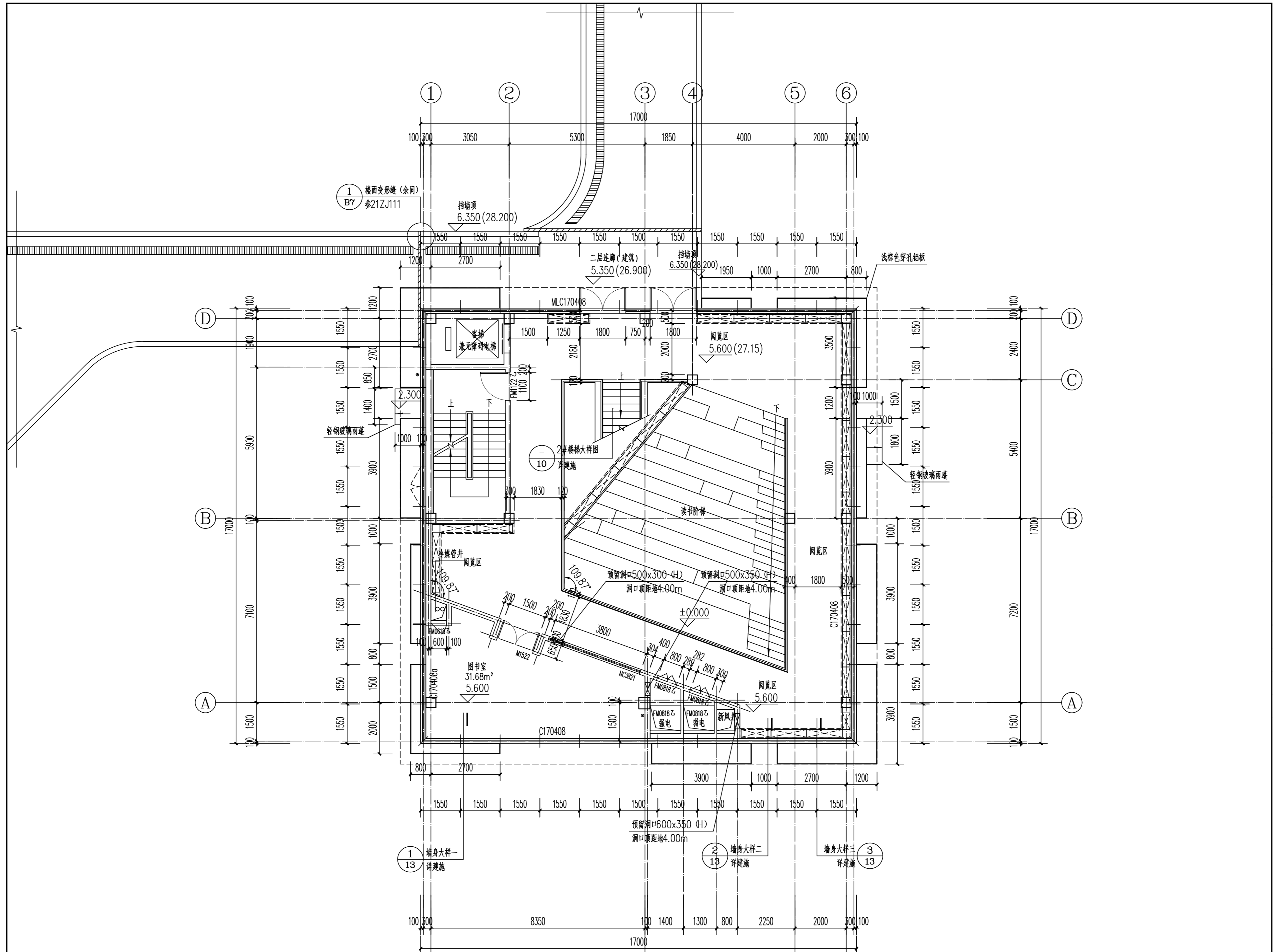
二层平面图 1:100 本层建筑面积 209.01 平方米
