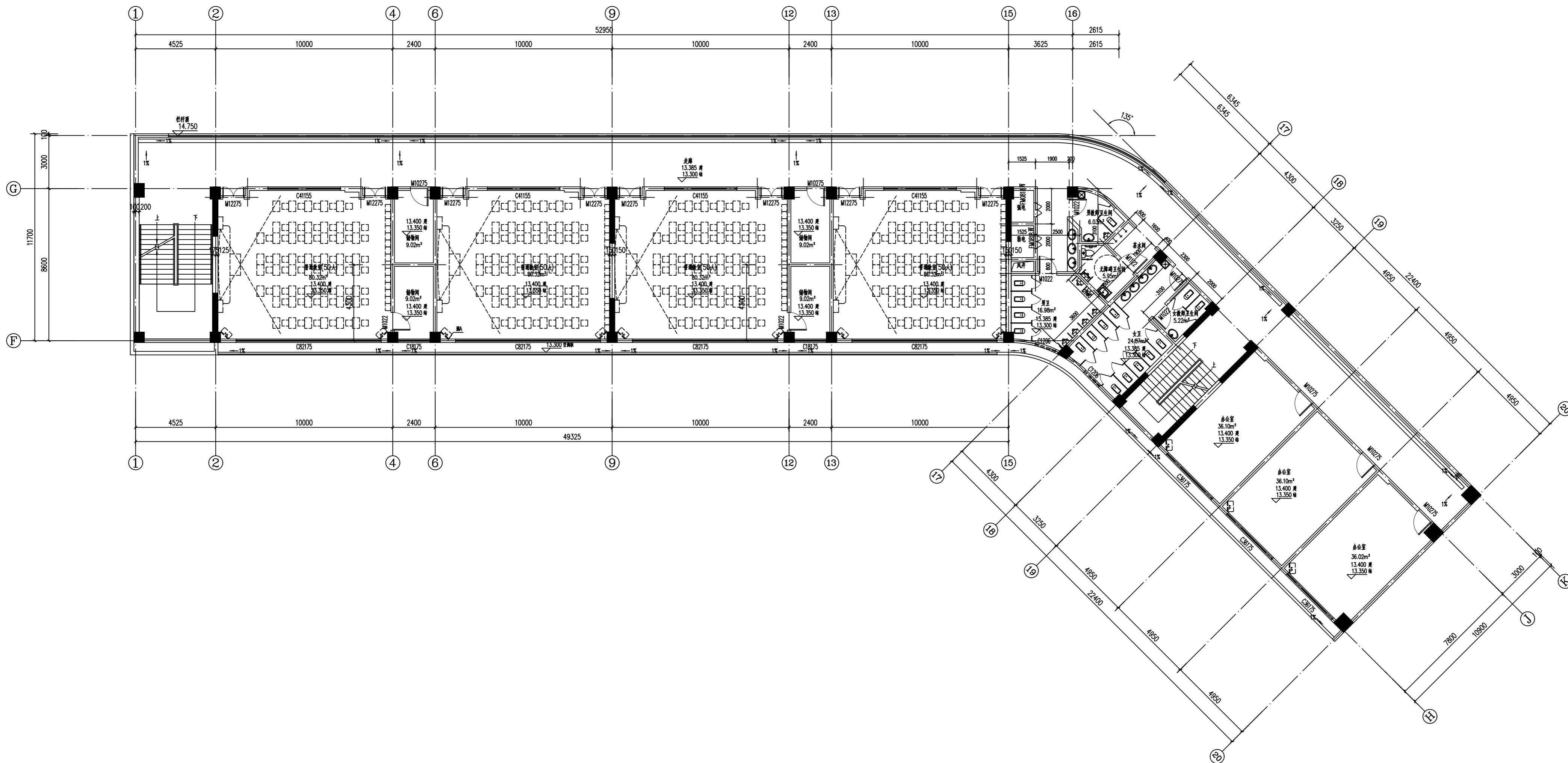
四层平面图 1:100 本层建筑面积: 924.32m²
