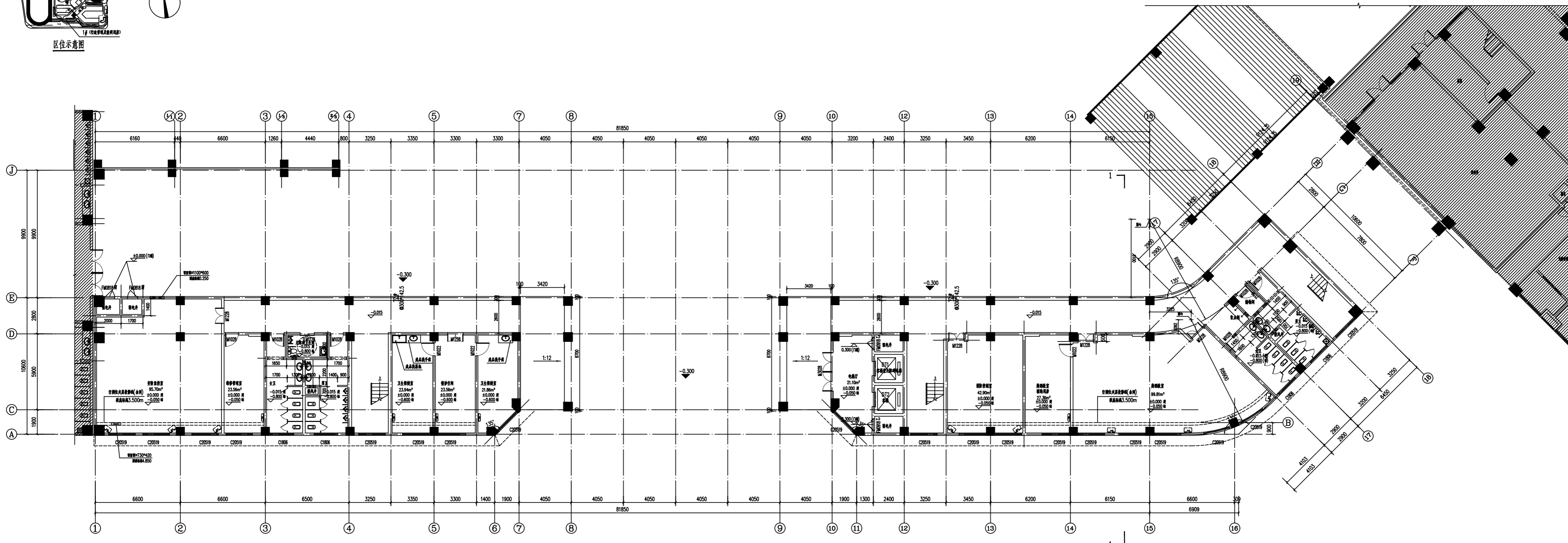
一层平面图 1:100
