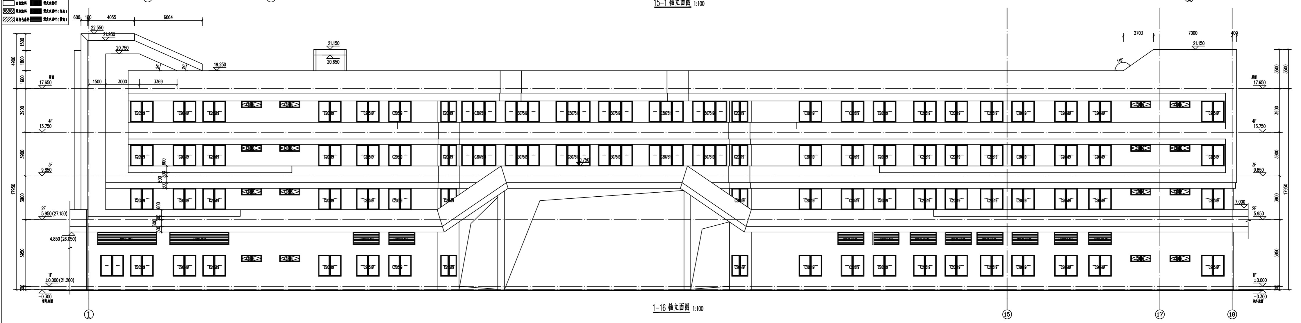
15-1 轴立面图 1:100
