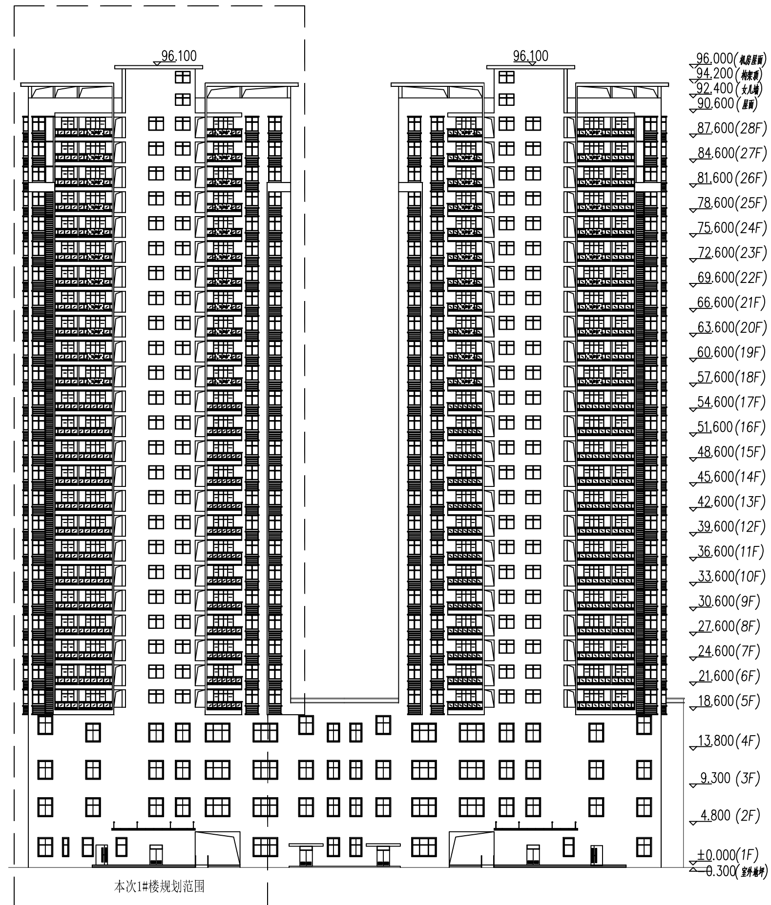
南立面图 1:350
