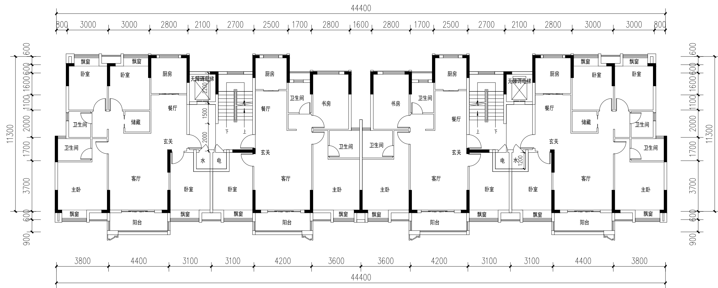
3#住宅二至七层平面图
