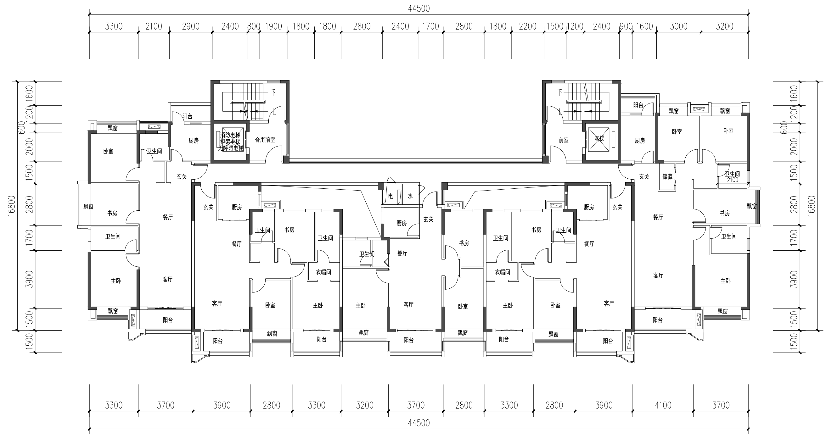
2#住宅四至二十层平面图
