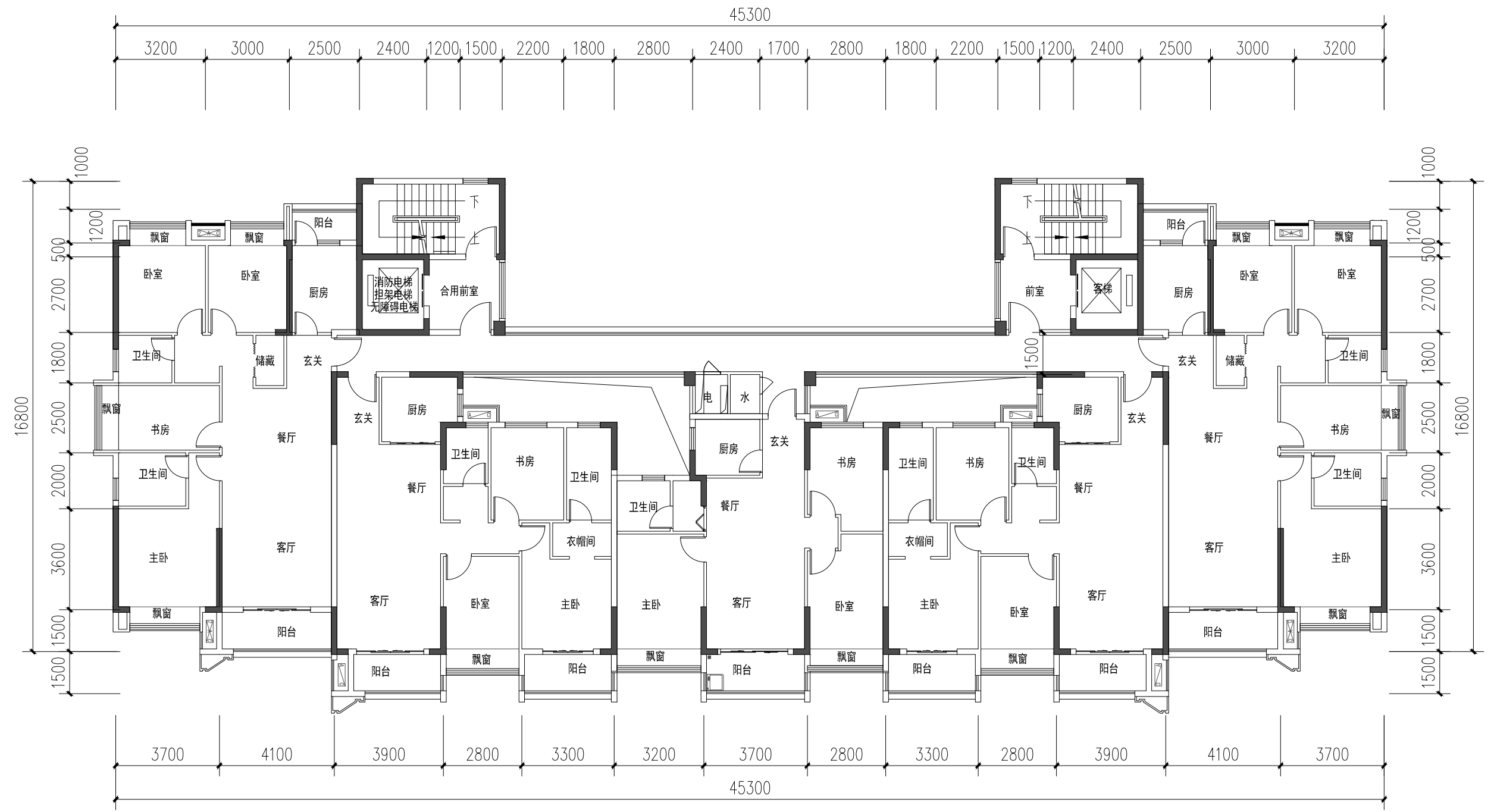
1#住宅四至二十五层平面图
