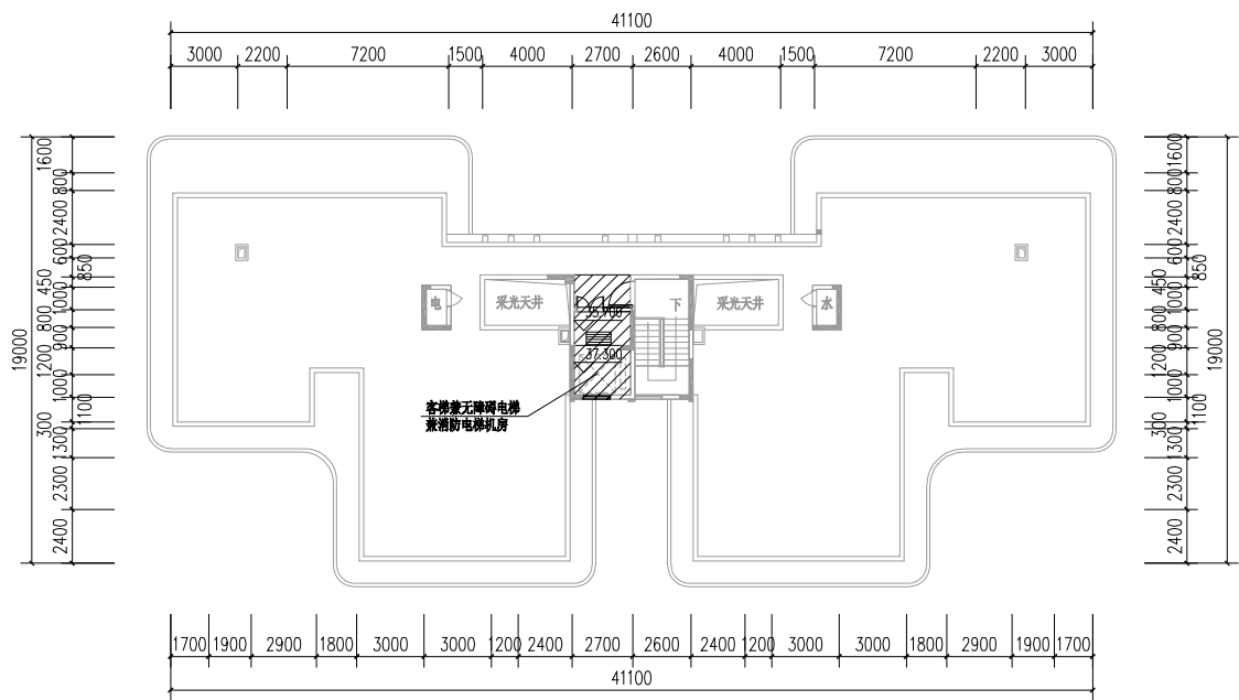
1#楼屋面平面图 1:250
