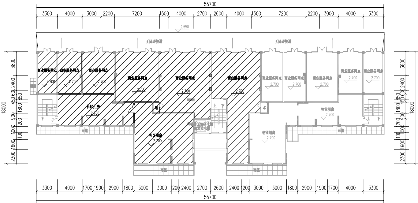
1#楼二层平面图 1:250
