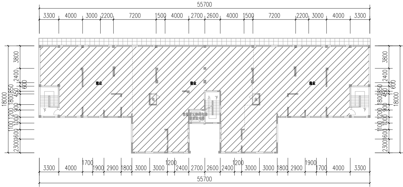
1#楼三层平面图 1:250
