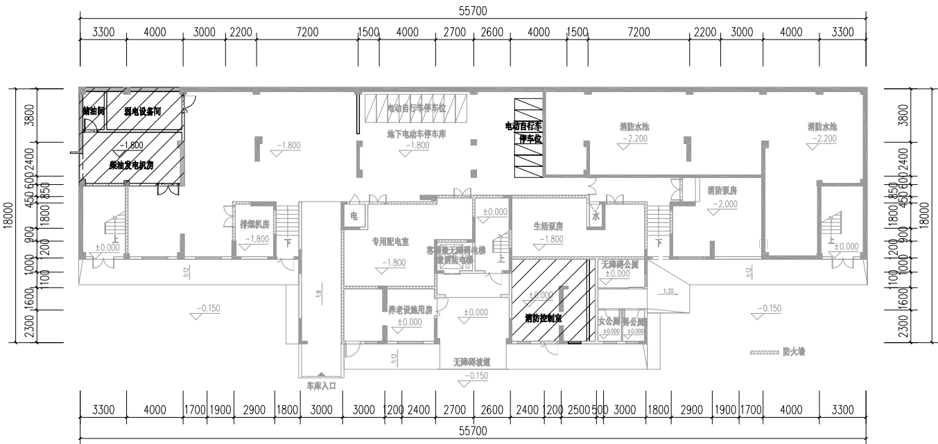
1#楼一层平面图 1:250 (局部为半地下室空间)
