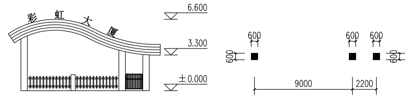
南立面图 1:200
